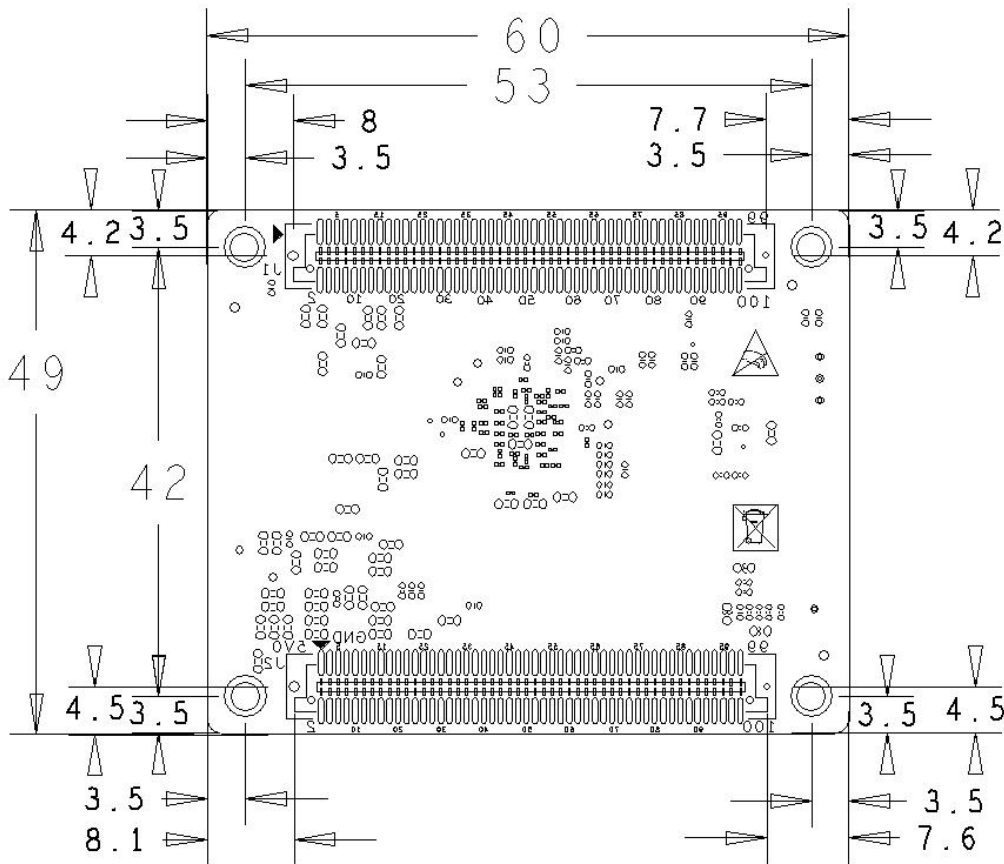
MYC-C8MMX-V2 Dimensions Chart
