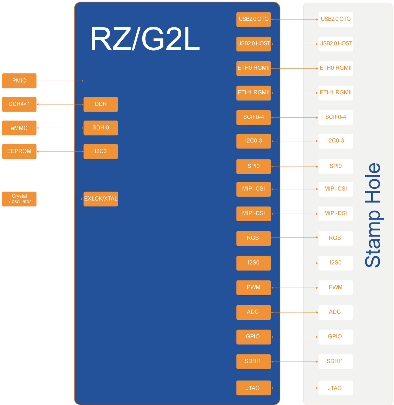
MYC-YG2LX SOM Function Block Diagram
