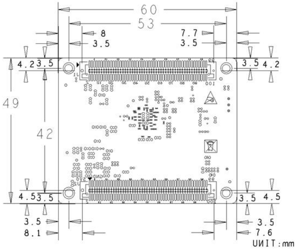
MYC-C8MMX-V2 Dimensions Chart
