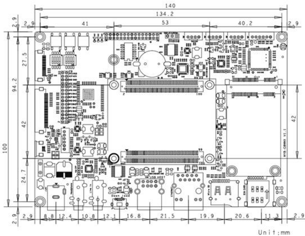
MYD-C8MMX-V2 Dimensions Chart
