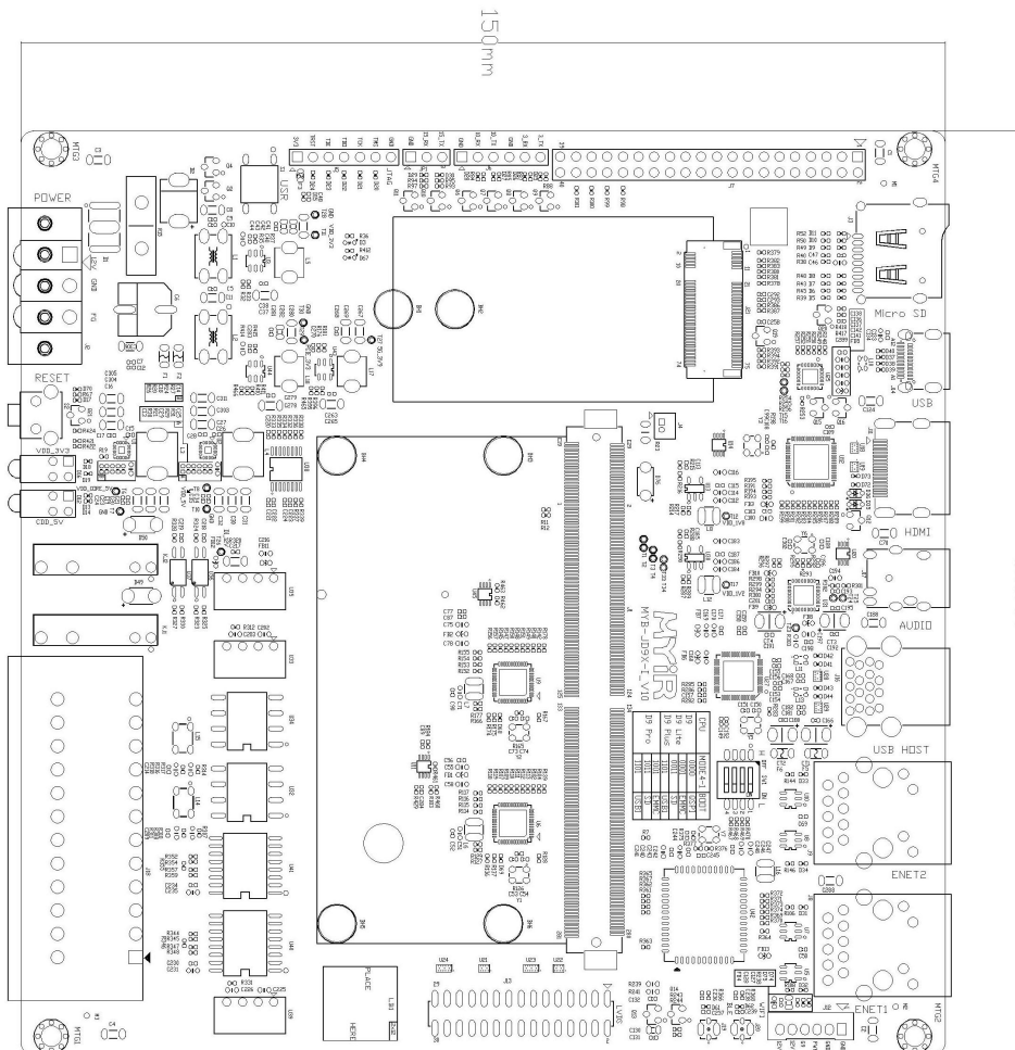
MYD-JD9360 Dimensions Chart
