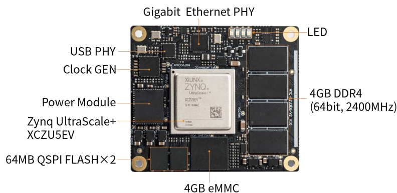
MYC-CZU3EG/4EV/5EV-V2 CPU Module
